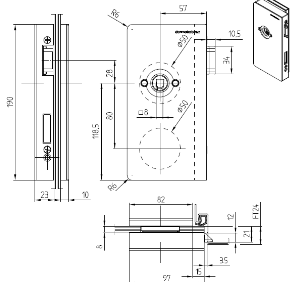
Zamek Junior Office
